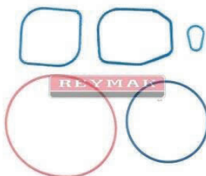
JUEGO DE LIGAS PARA TAPA DE ÁRBOL DE LEVAS MOTOR DETROIT DIESEL SERIE 60
