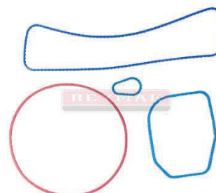
JUEGO DE LIGAS PARA ÁRBOL DE LEVAS MOTOR DETROIT "SERIE 60" TIPO NUEVO
